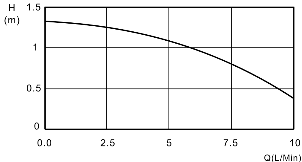
Рис.2. Расходно-напорная характеристика насоса.
